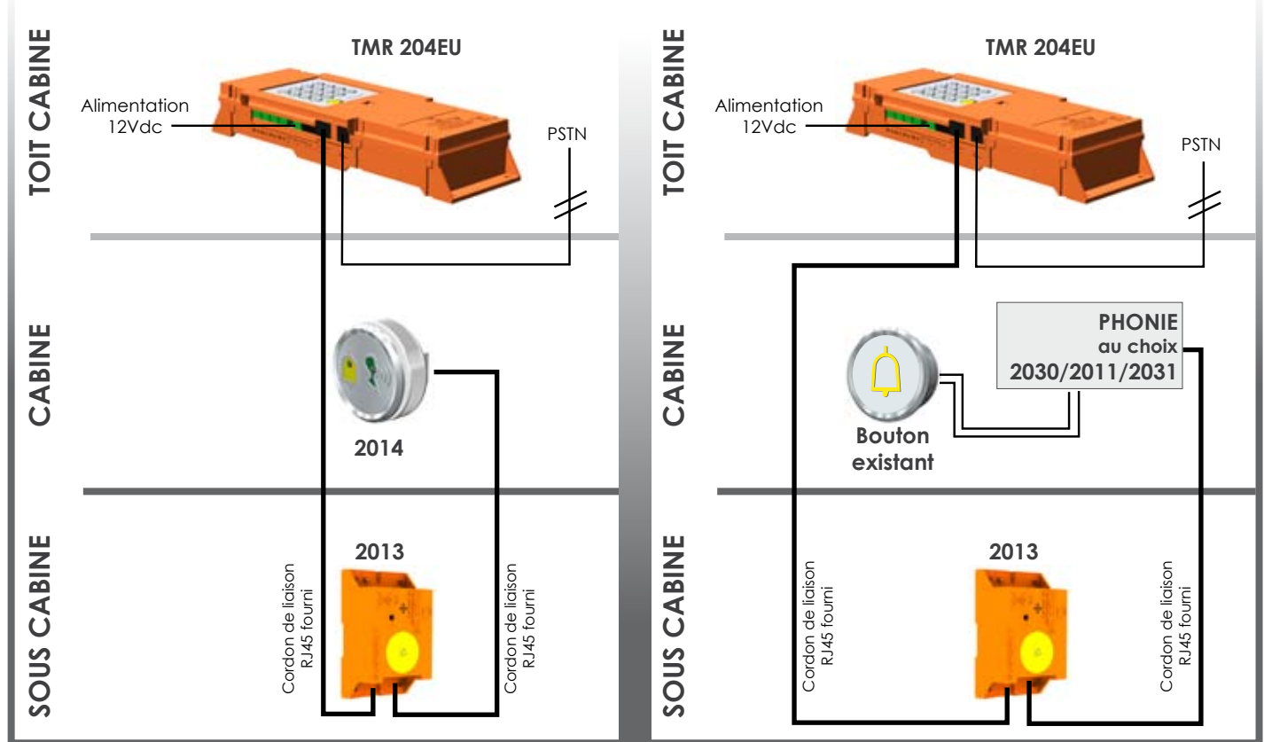
PACK TRIPHONIE TMR204EU + bouton cabine 2014 + module sous cabine 2013
