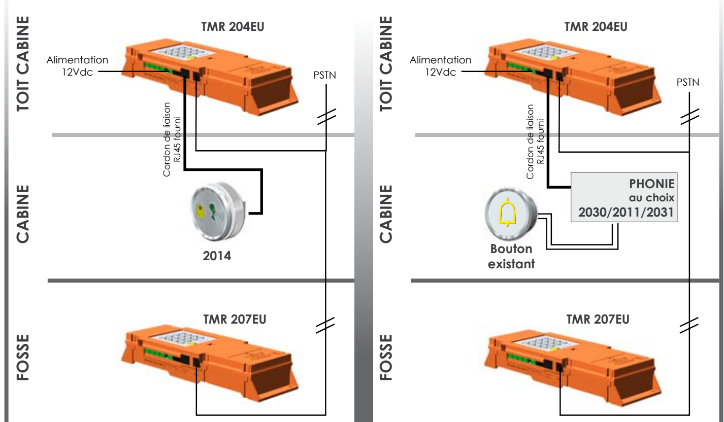
PACK TRIPHONIE TMR204EU + bouton cabine 2014 + module fond de fosse TMR 207EU
