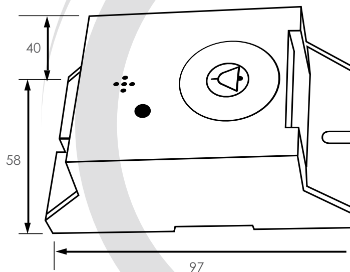
PLAN D'ENCOMBREMENT
